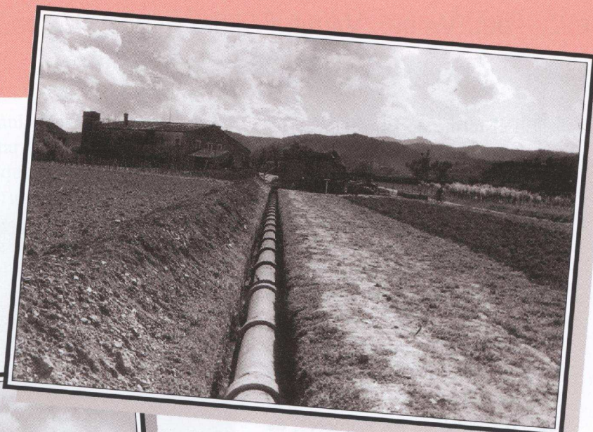
Regadiu de Juià, canonada d'impulsió, últim tram d'arribada al dipòsit distribuïdor, en fase de construcció, l'any 1959.
